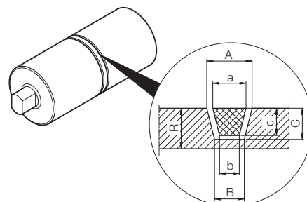
Fig.: V-grooved lagging
